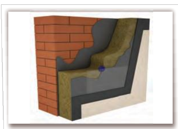
Wand-Wärmedämmsystem
