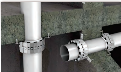
Conducte metalice neizolate/izolate cu materiale combustibile
